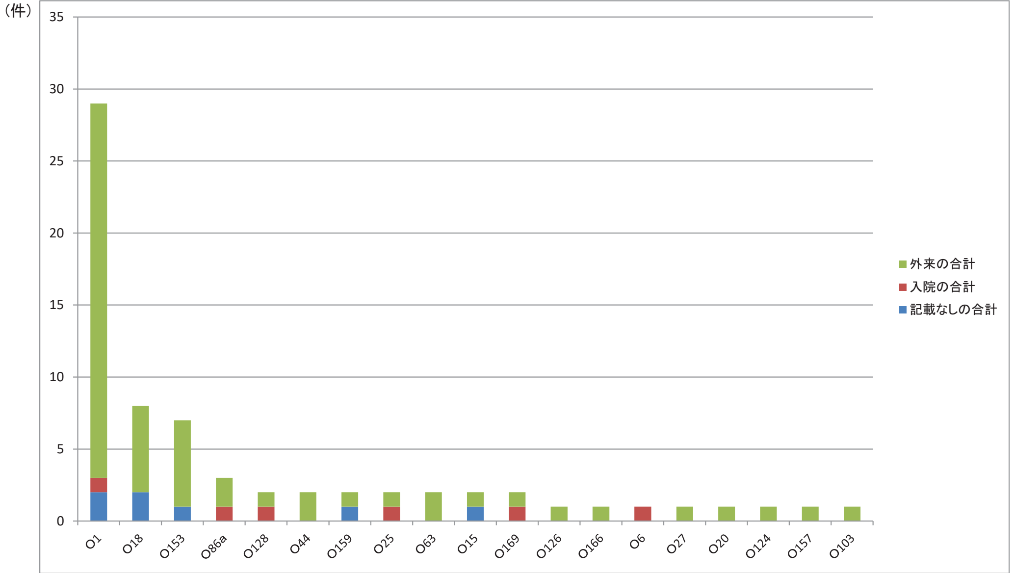
【病原大腸菌 型別】細菌検出状況 2024年06月
