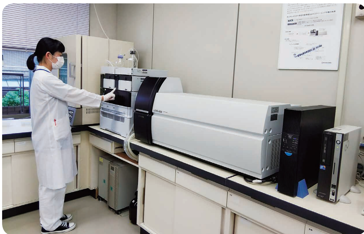
先天性代謝異常検査室の様子(タンデム型質量分析計)
