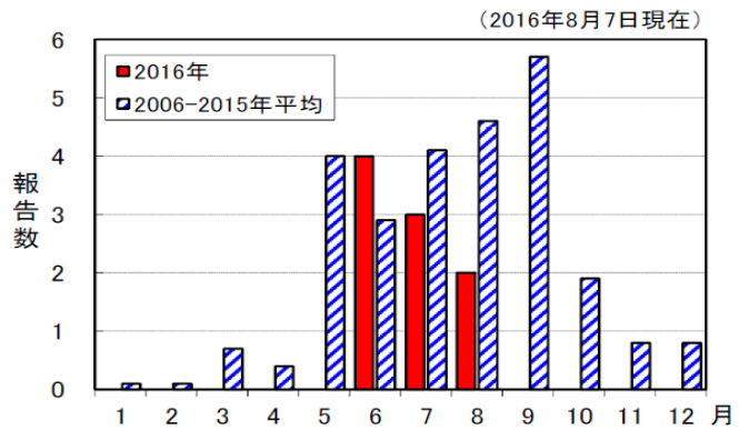
広島市における腸管出血性大腸菌感染症の月別報告数
